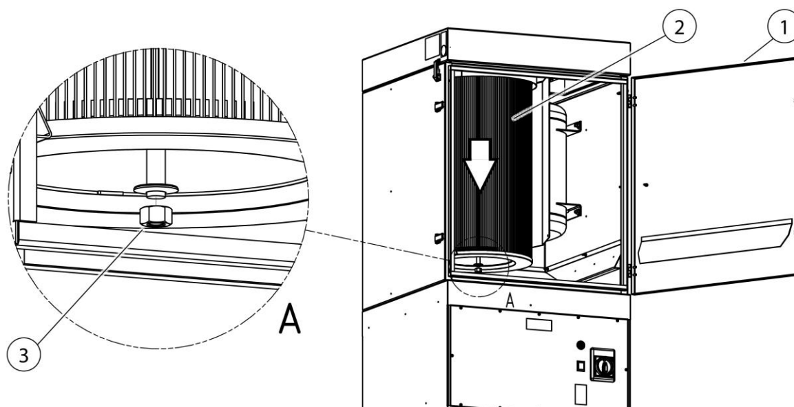
Рис. 9: Замена фильтра
