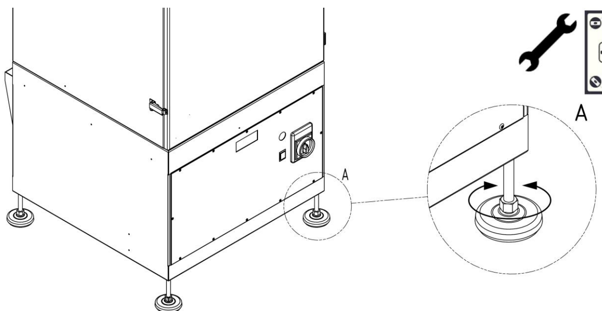
Рис. 2: Установка устройства
