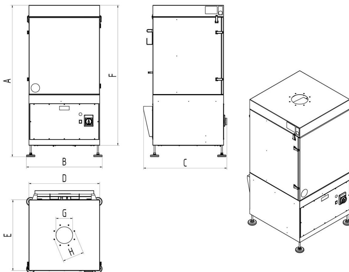
Рис. 13: Габаритный чертеж
