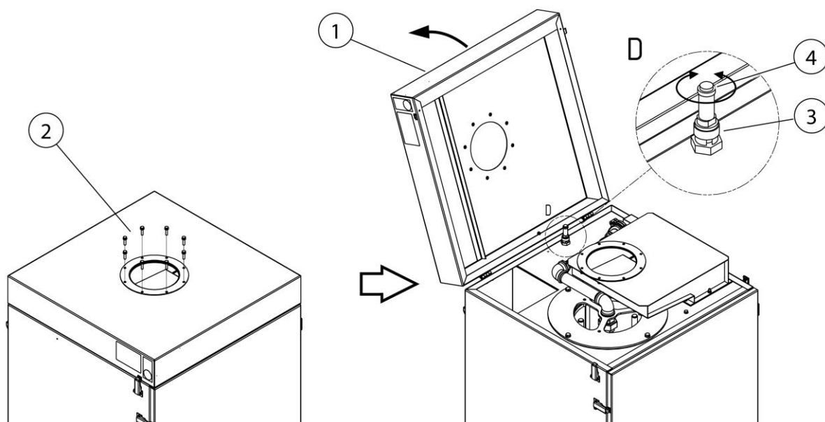
Рис. 12: Доступ к предохранительному клапану сжатого воздуха
