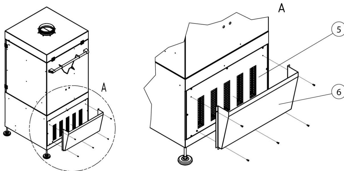
Рис. 4: Монтаж выпускного блока
