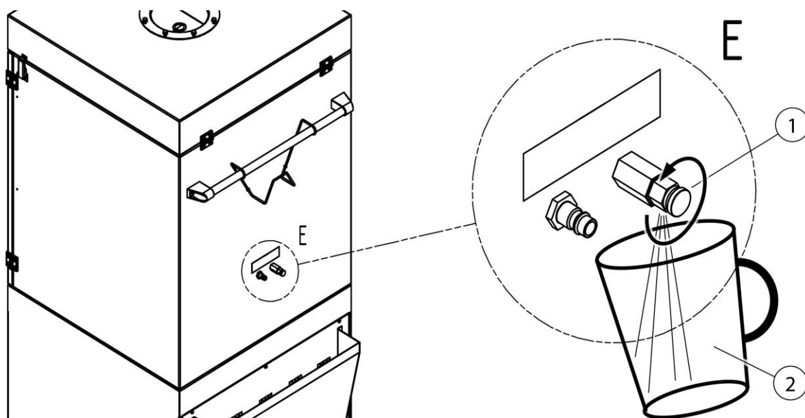
Рис. 8: Слив конденсата
